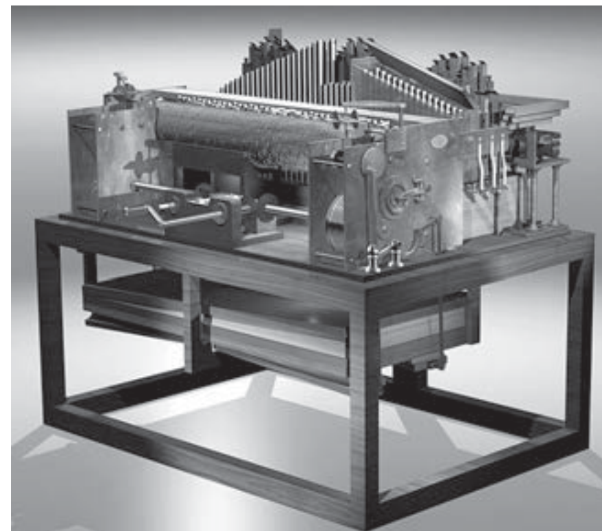
Музыкальный механизм Механического оркестра. Автор компьютерного моделирования П. А. Скобликов
